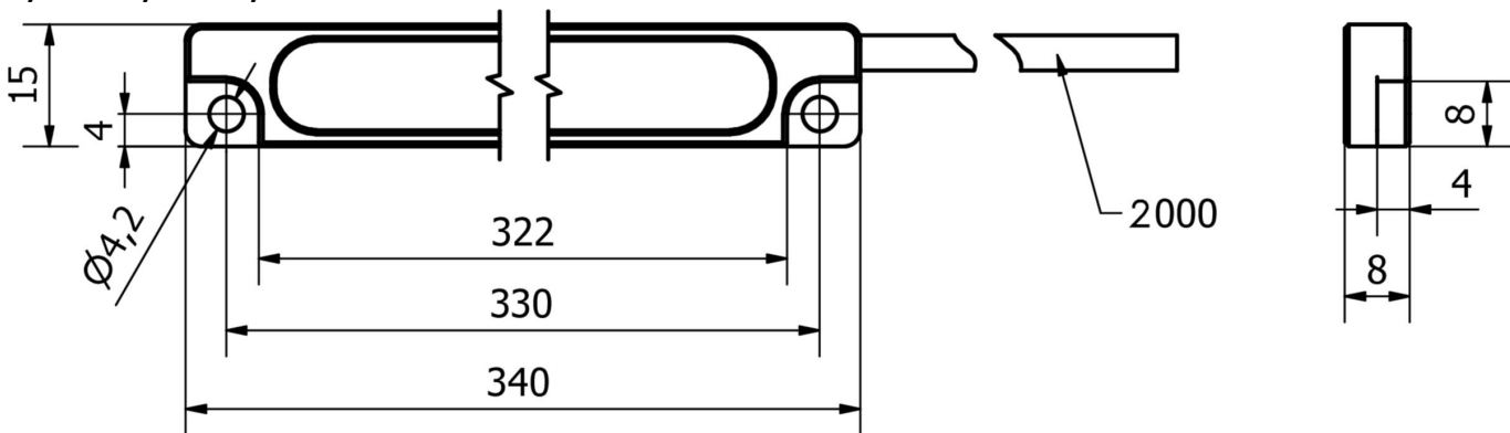
Rysunek wymiarowy
