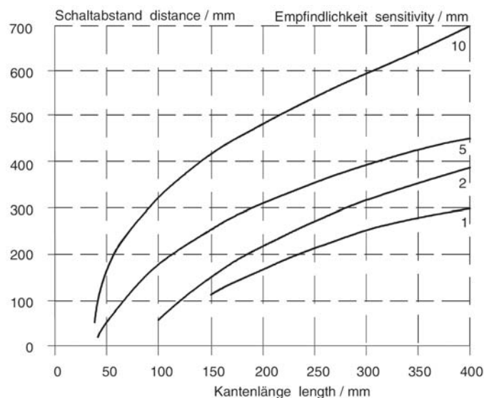
Bild 4: Ansprechdiagramm
