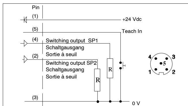
Wiring/Anschlüsse/Raccordement électrique
