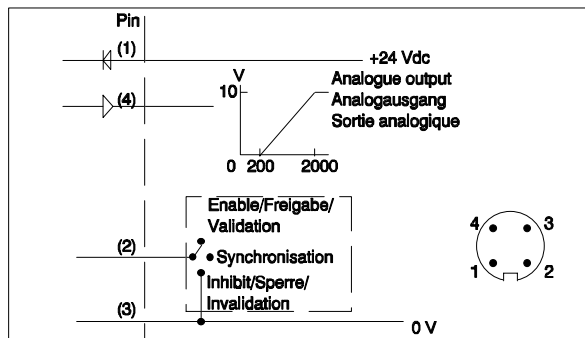
Wiring/Anschlüsse/Raccordement électrique
