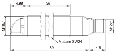
Maßskizze Sender:
