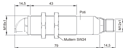
Maßskizze Empfänger
