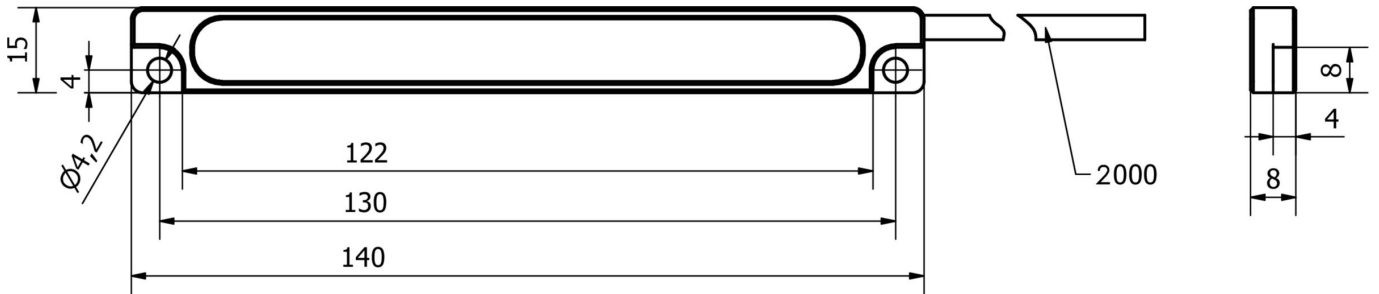
Rysunek wymiarowy
